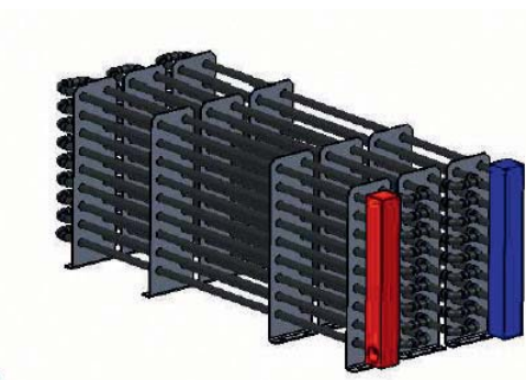
Echangeur de chaleur pour récupérer l'énergie en sortie de STEP (Source RWB)
